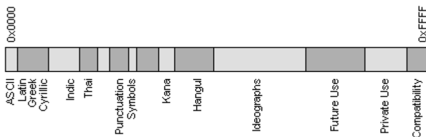
Рис. 9.1. Структура UNICODE.
